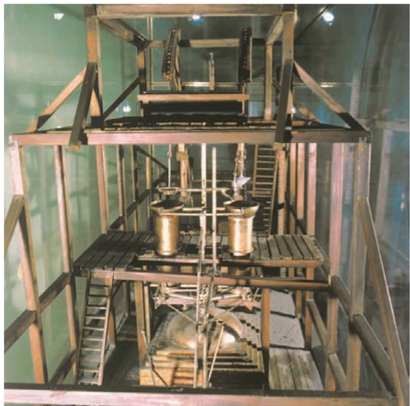
Макет паровой машины И. Ползунова
